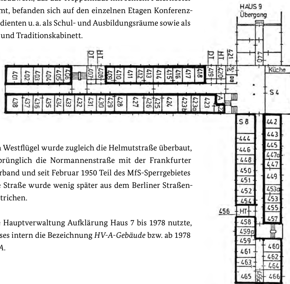
↑ Abb. 45: Grundriss von Haus 7 aus dem Jahr 1986. Man erkennt den langen Nord- und Westflügel, der kurze Ostflügel führt als Übergang zu Haus 9.
